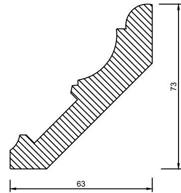
Sez.A-A
