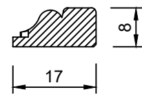
Sez. A-A
