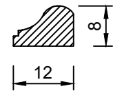
Sez. A-A
