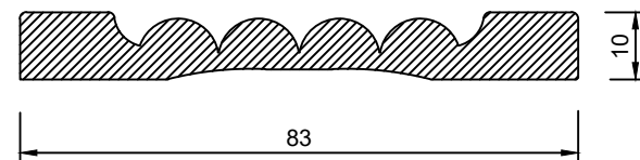
Sez.A-A
