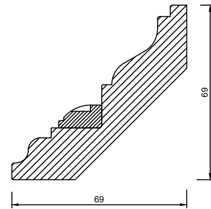
Sez.A-A
