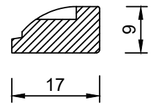
Sez.A-A
