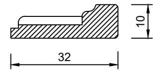
Sez.A-A
