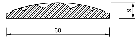
Sez.A-A
