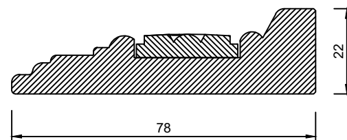
Sez.A-A
