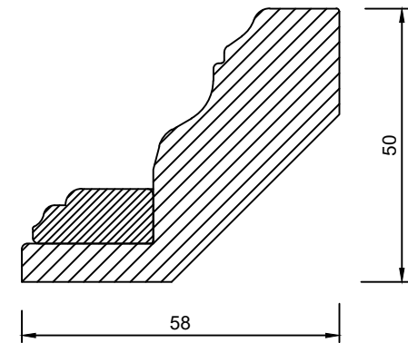
Sez.A-A
