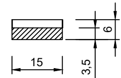
Sez.A-A
