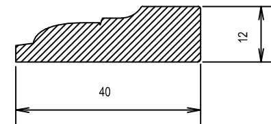
Sez.A-A
