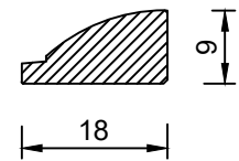
Sez.A-A
