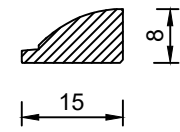
Sez.A-A
