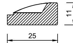
Sez.A-A
