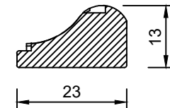
Sez. A-A
