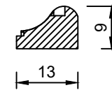
Sez. A-A
