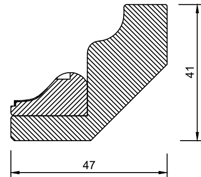
Sez.A-A
