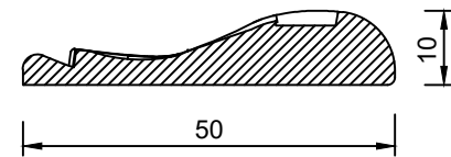
Sez.A-A
