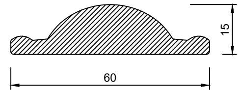
Sez.A-A
