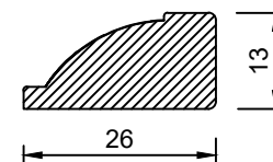
Sez.A-A
