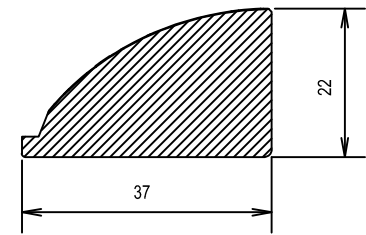
Sez.A-A
