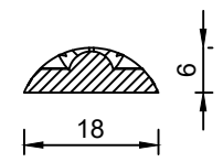
Sez.A-A
