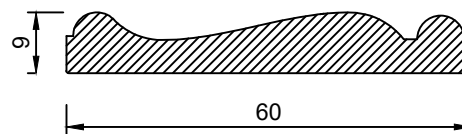
Sez.A-A
