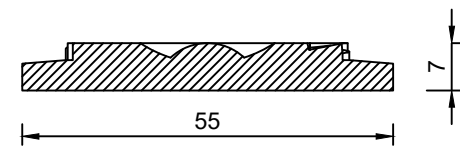
Sez.A-A
