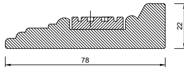
Sez.A-A
