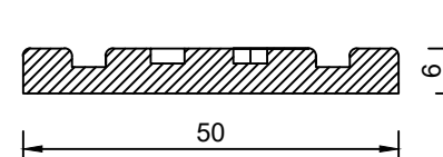
Sez.A-A
