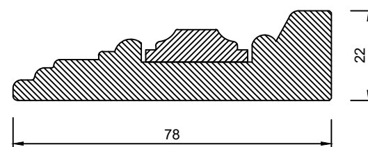
Sez.A-A
