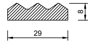
Sez.A-A
