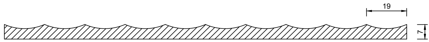
Sez. A-A
